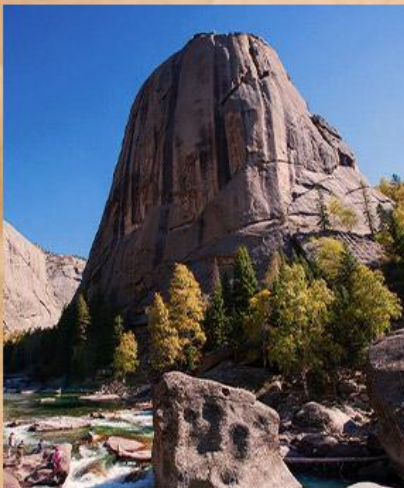
可可托海世界地质公园
